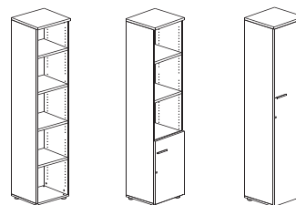
2030 x 450 x 425
